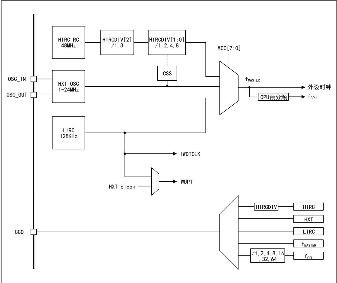
图4 APM32F003F6UX 系列时钟树
