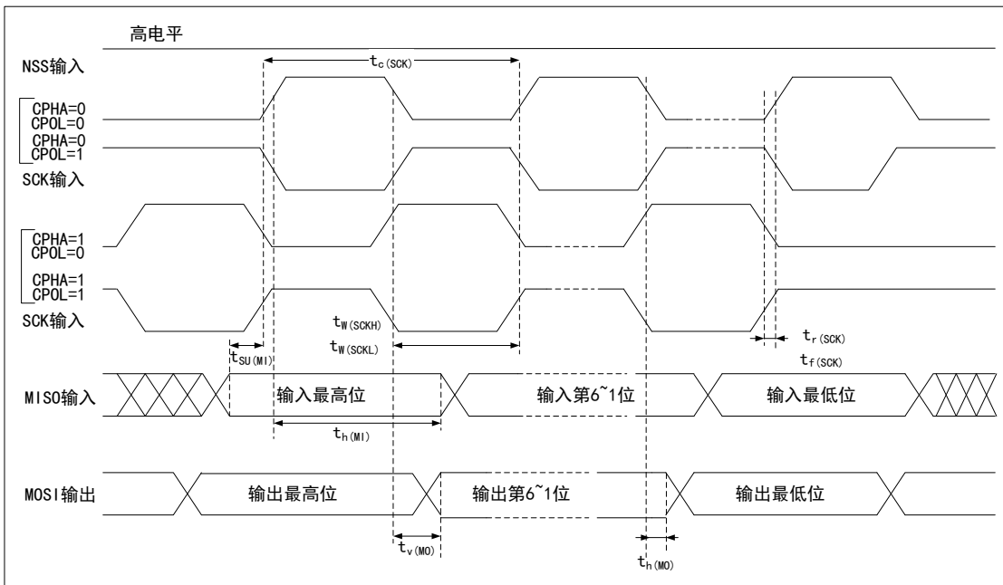
图11 SPI 时序图—主模式
