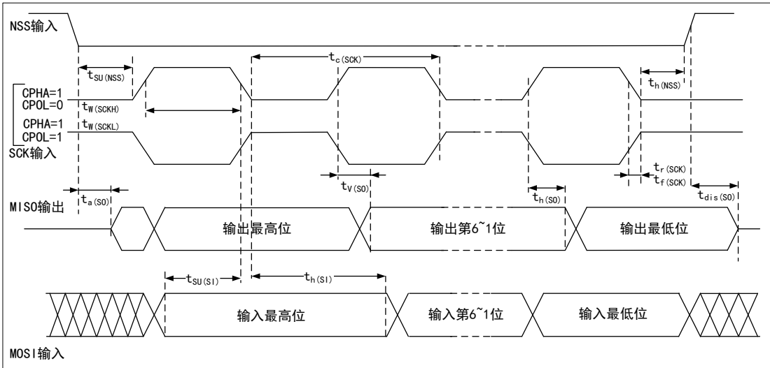
图10 SPI 时序图—从模式和 CPHA=1
