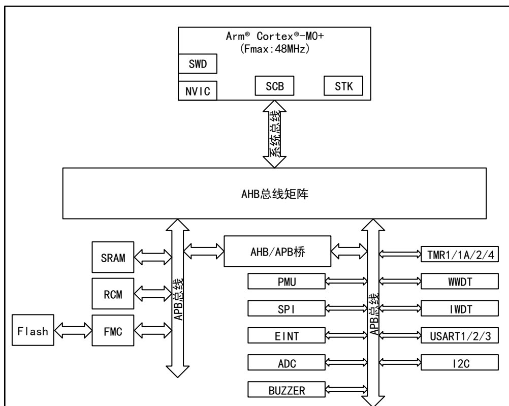
图2 APM32F003F6UX 系列系统框图
