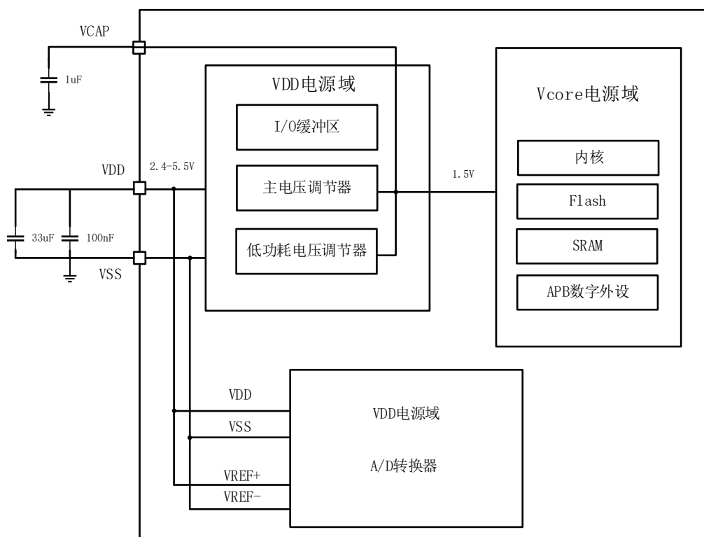
图5 电源方案
