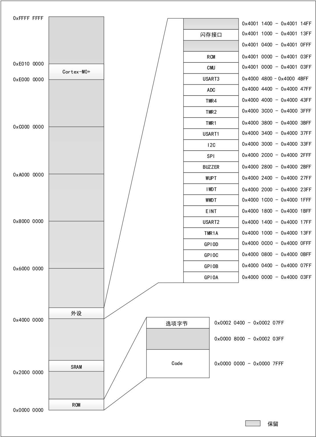
图3 APM32F003F6UX 系列地址映射图
